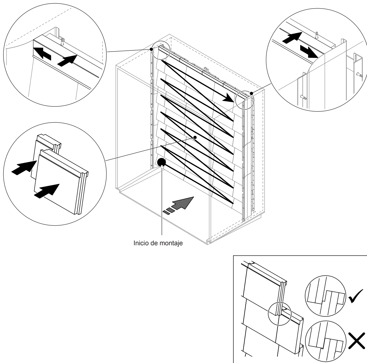
Fig. 10: Montaje de las placas cerámicas
