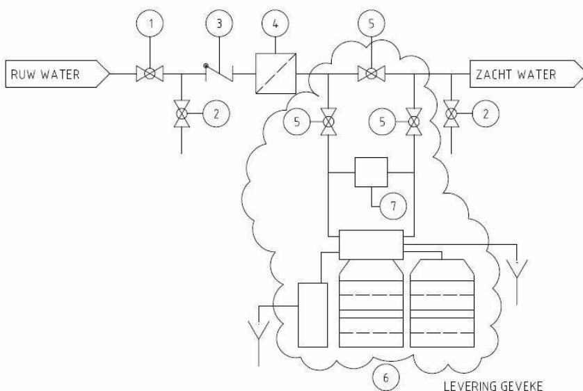
Installatieschema CondairSoft 010D t/m 070D
