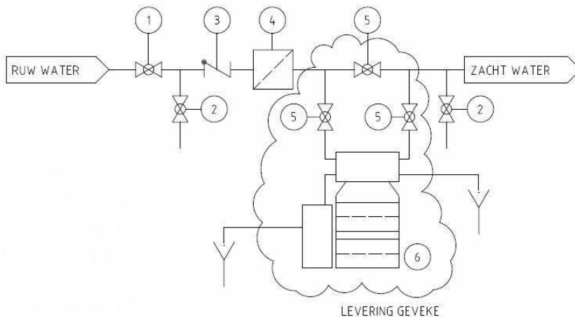
Installatieschema CondairSoft 010D t/m 070D
