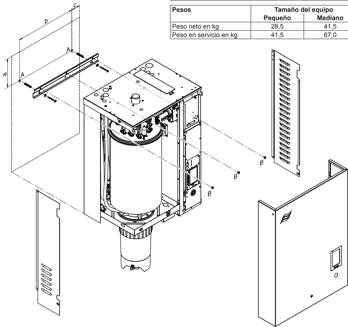
Fig. 13: Resumen del montaje de equipos individuales pequeños y medianos con carril de montaje
