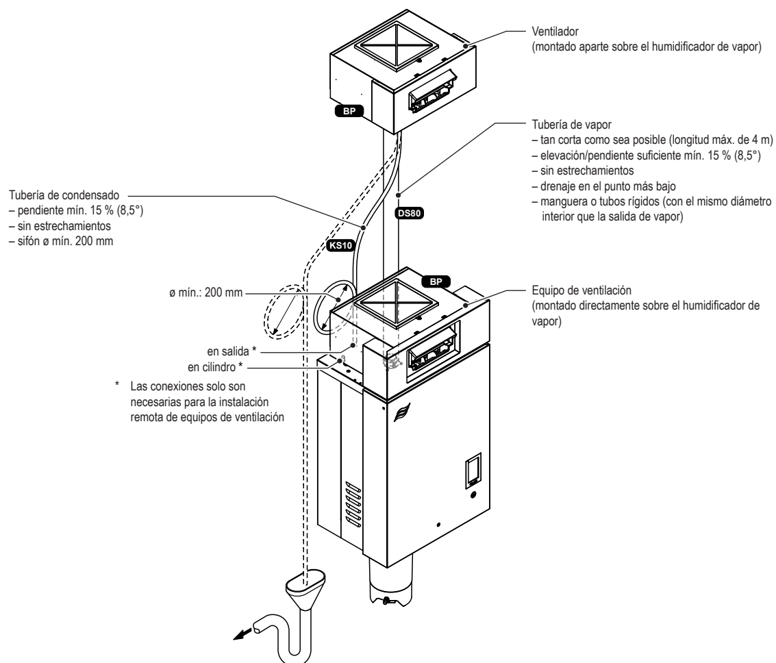
Fig. 16: Resumen de la instalación de vapor, humidificación ambiental directa
