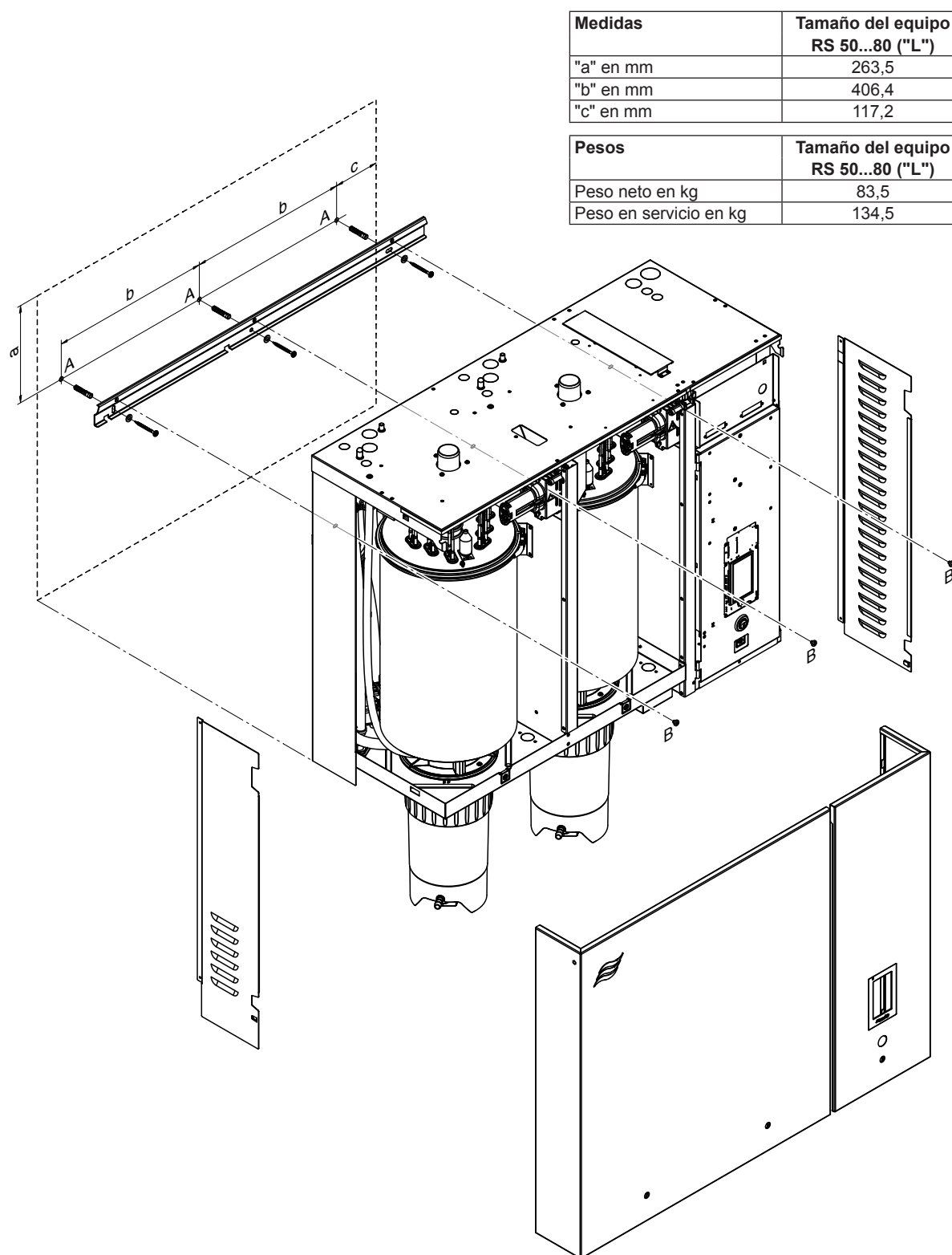
Fig. 14: Resumen del montaje de equipos individuales grandes con carril de montaje
