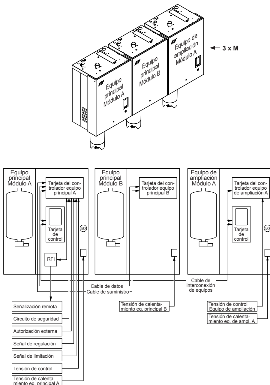
Fig. 4: Resumen de los sistemas interconectados (3 x "M")
