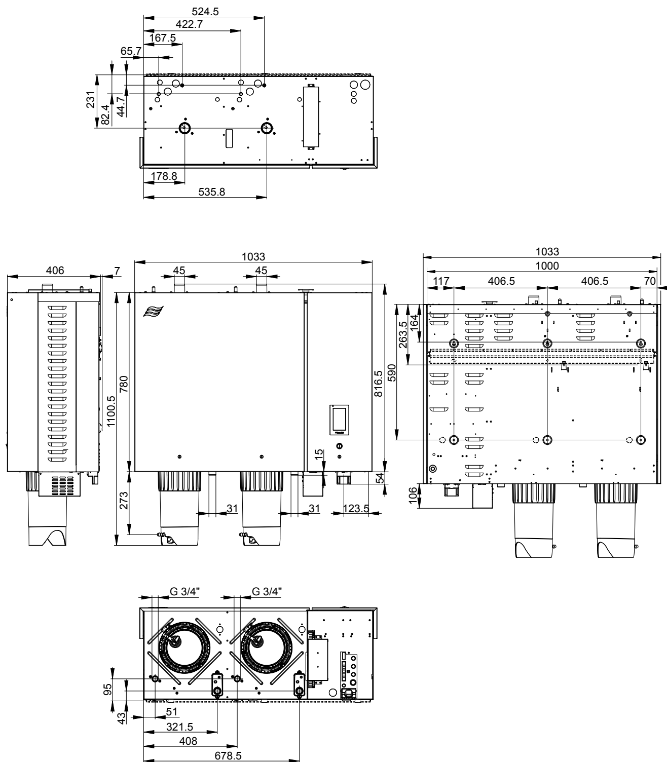
Fig. 36: Figura de dimensiones del equipo "L" (dimensiones en mm)
