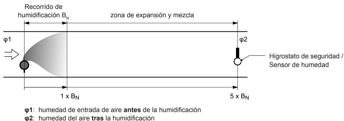
Fig. 17: Recorrido de humidificación " B_N "
