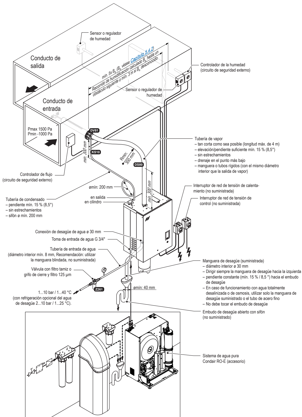
Fig. 8: Instalación típica para la humidificación de conducto
