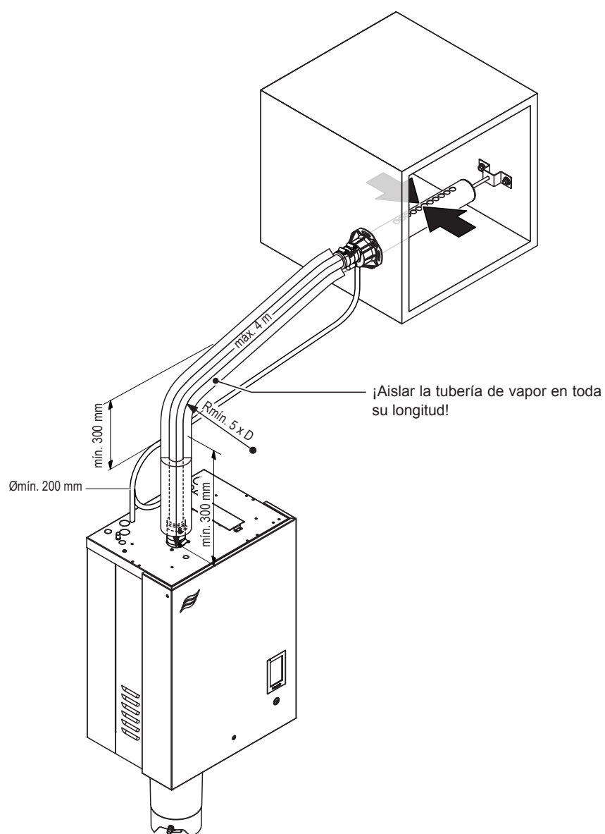
Fig. 20: Tubería de vapor con tubos rígidos y aislamiento
