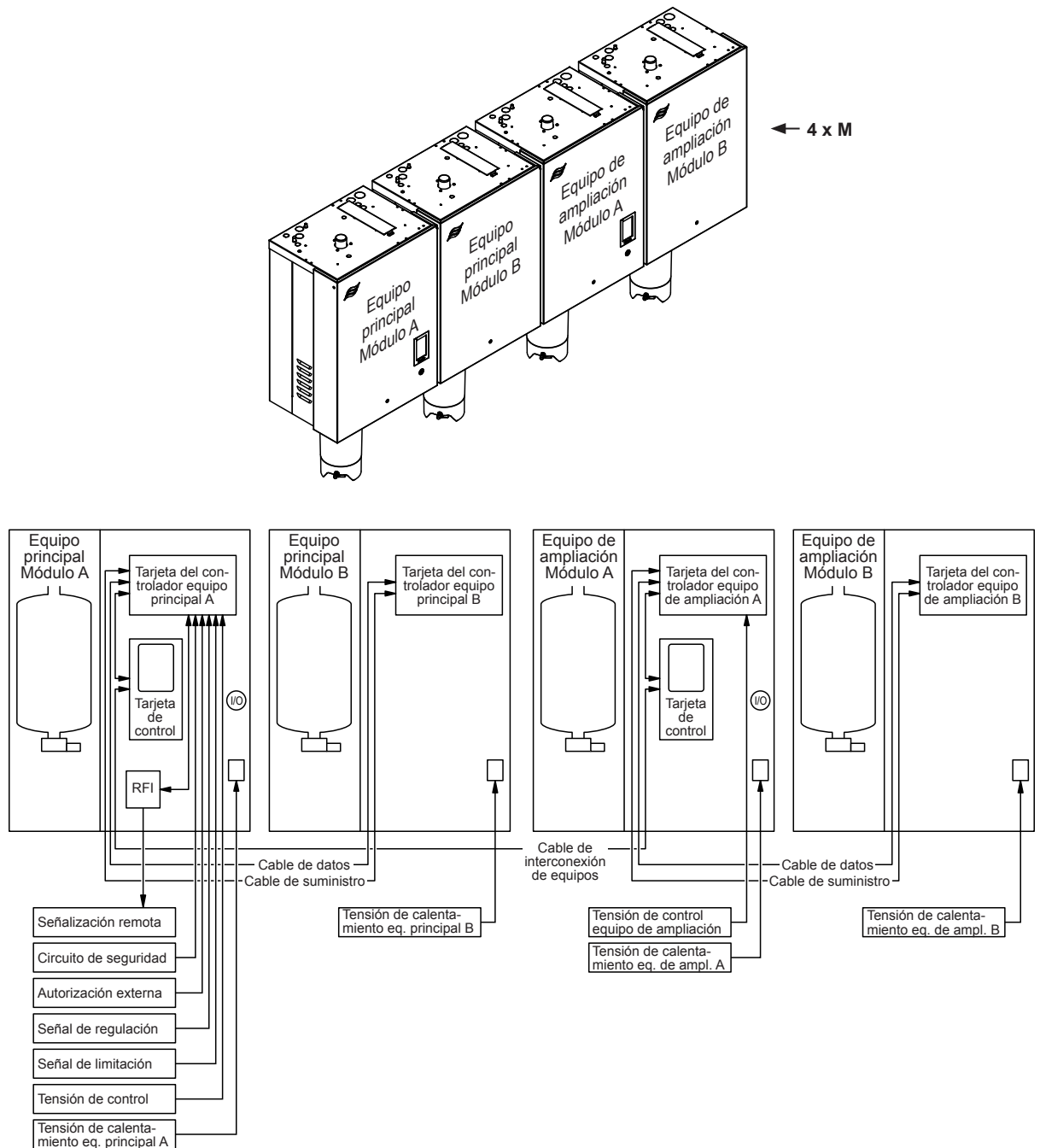
Fig. 5: Resumen de los sistemas interconectados (4 x "M")
