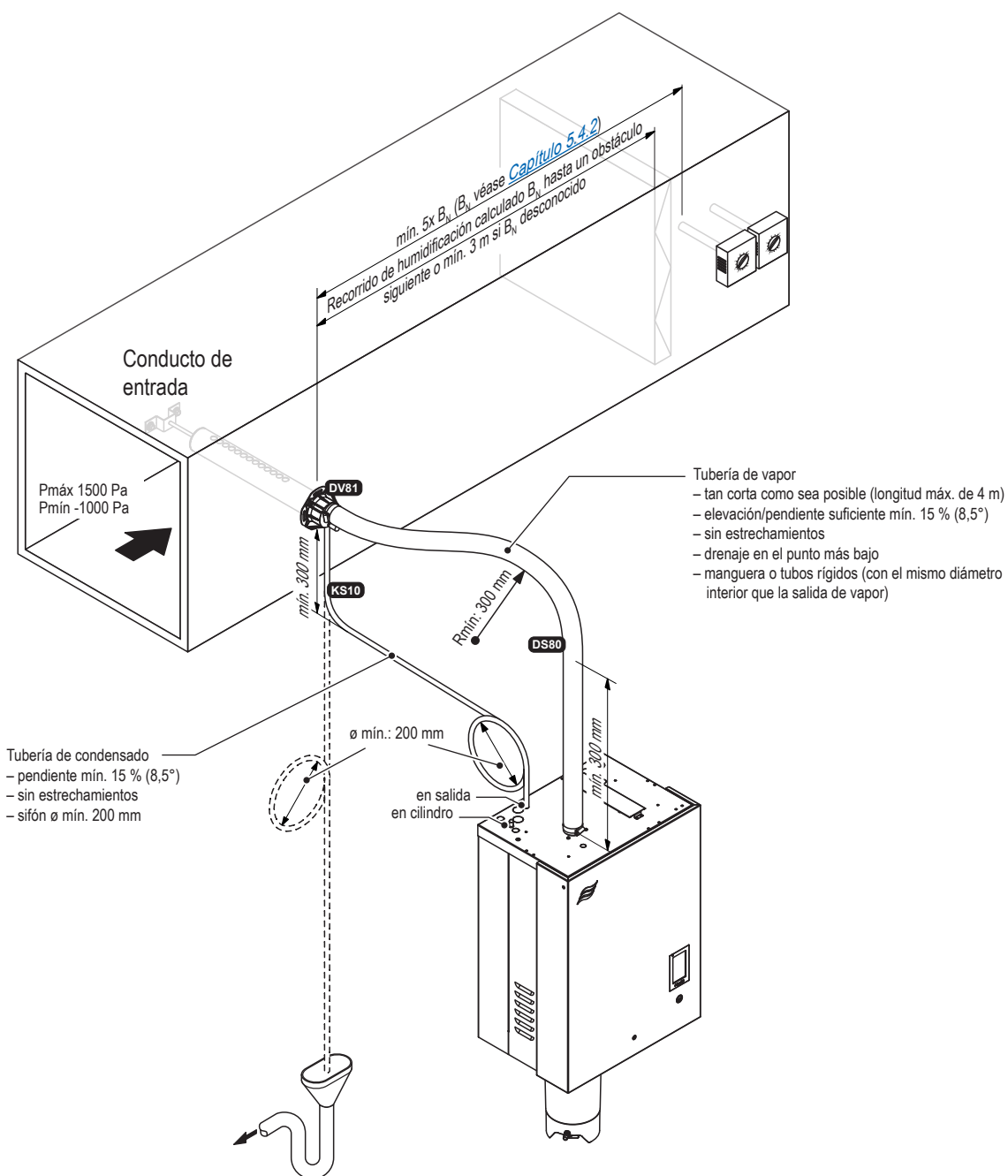
Fig. 15: Resumen de la instalación de vapor, humidificación de conducto
