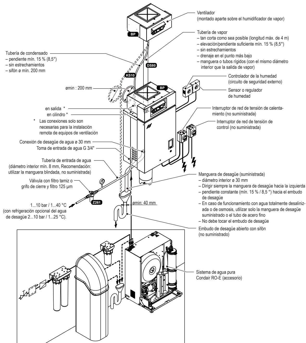
Fig. 9: Instalación típica para la humidificación directa del ambiente
