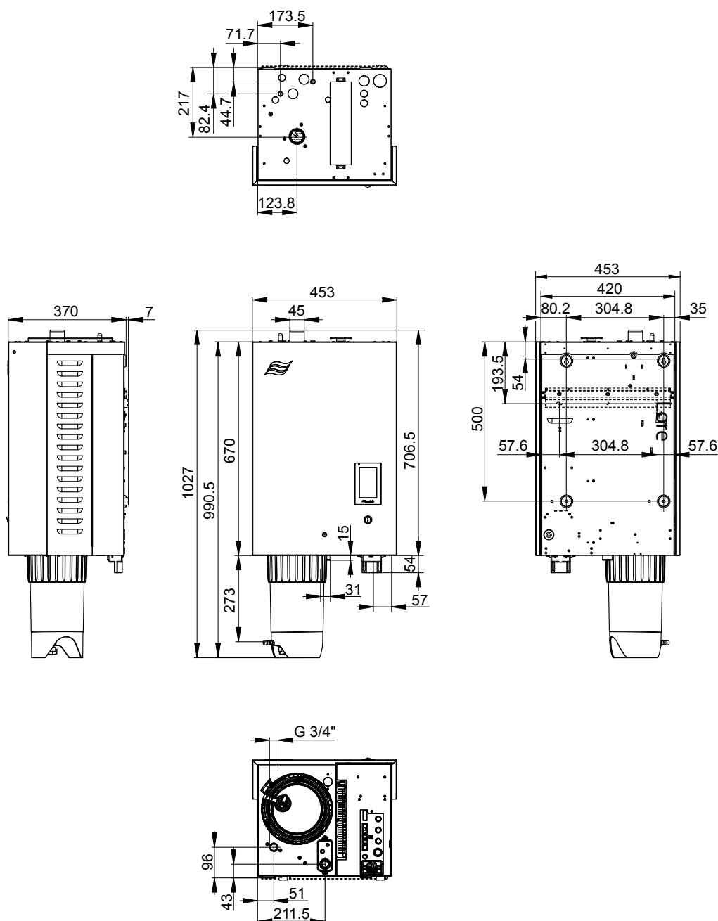
Fig. 34: Figura de dimensiones del equipo "S" (dimensiones en mm)
