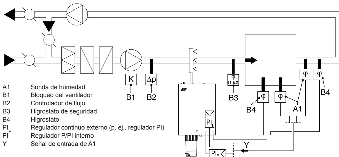
Fig. 25: Sistema 1 – Regulación de la humedad ambiental
