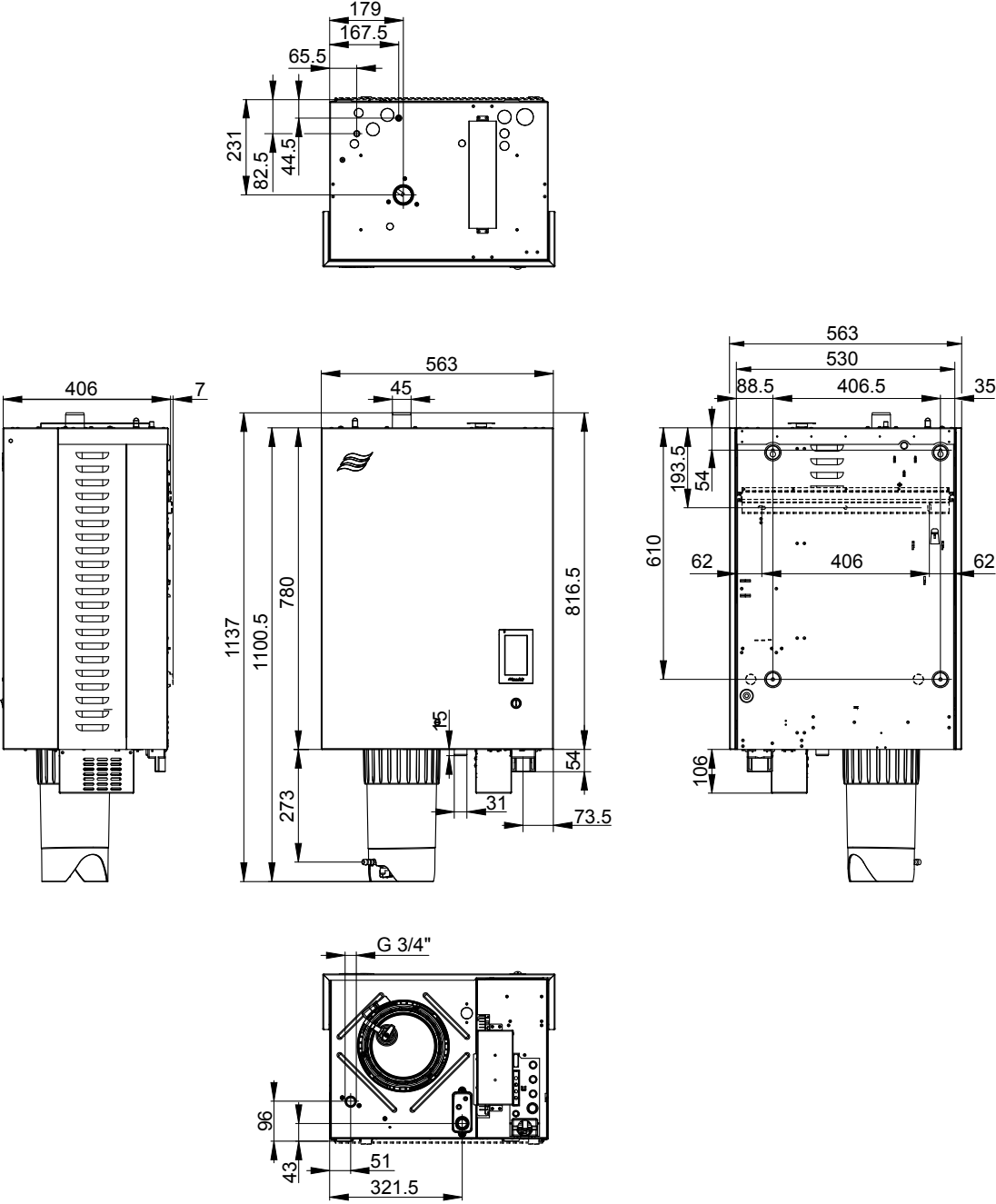
Fig. 35: Figura de dimensiones del equipo "M" (dimensiones en mm)
