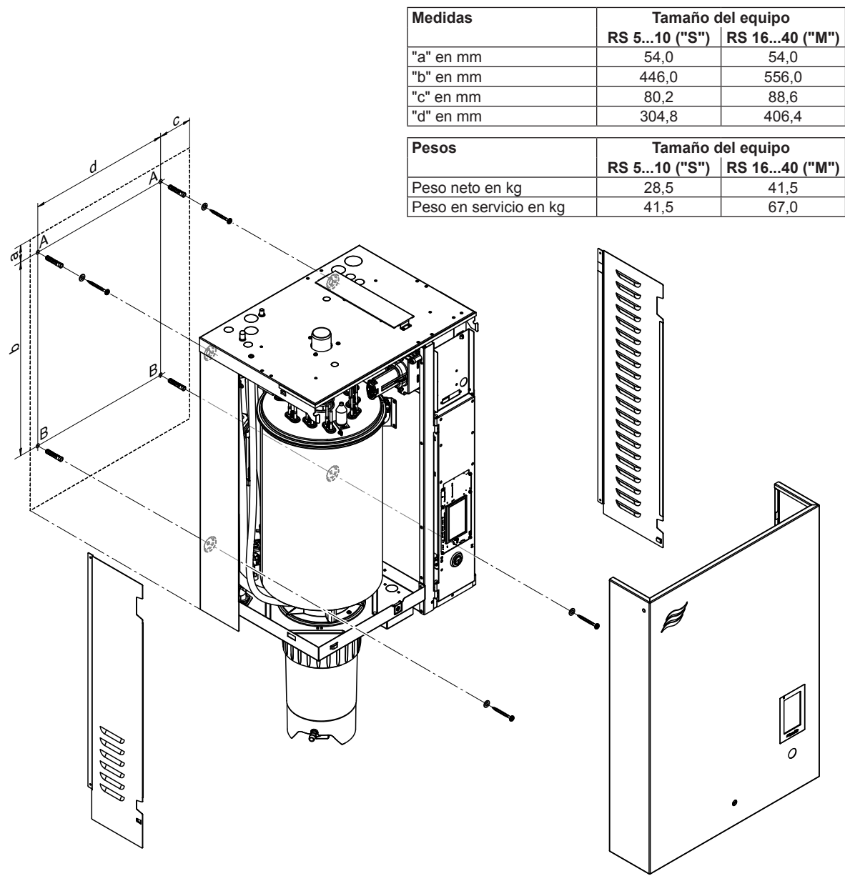
Fig. 11: Resumen del montaje estándar de equipos individuales pequeños y medianos
