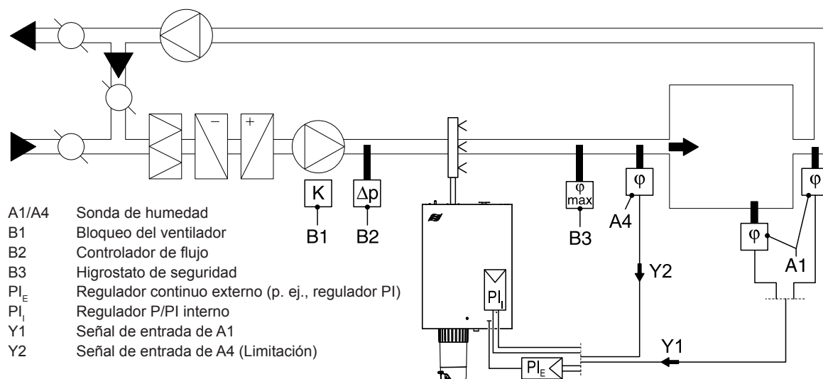
Fig. 26: Sistema 2 – Regulación de la humedad ambiental con limitación continua de la humedad de entrada
