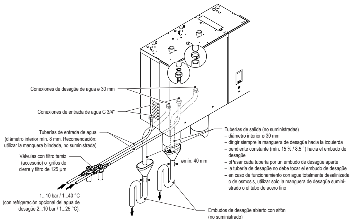
Fig. 23: Resumen de la instalación de agua para equipos individuales grandes ("L")
