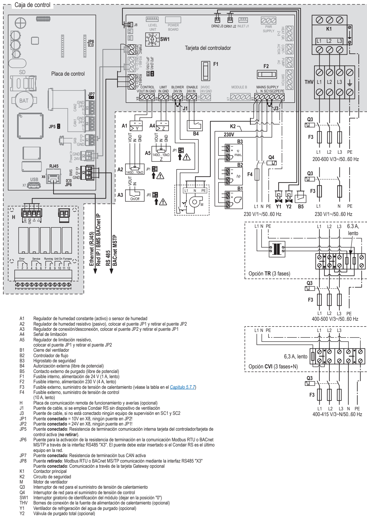
Fig. 28: Esquema eléctrico del Condair RS: equipos individuales "S" y "M" (5...40 kg/h)
