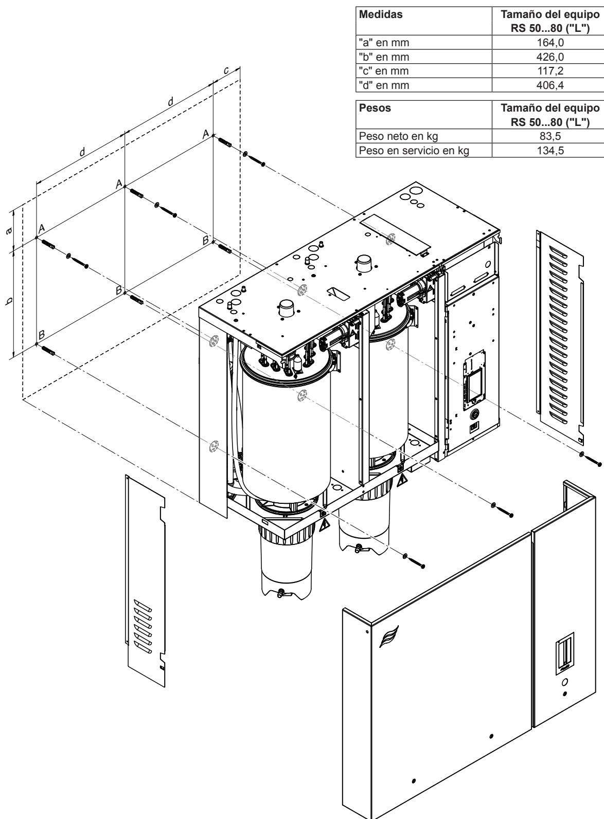
Fig. 12: Resumen del montaje estándar de equipos individuales grandes
