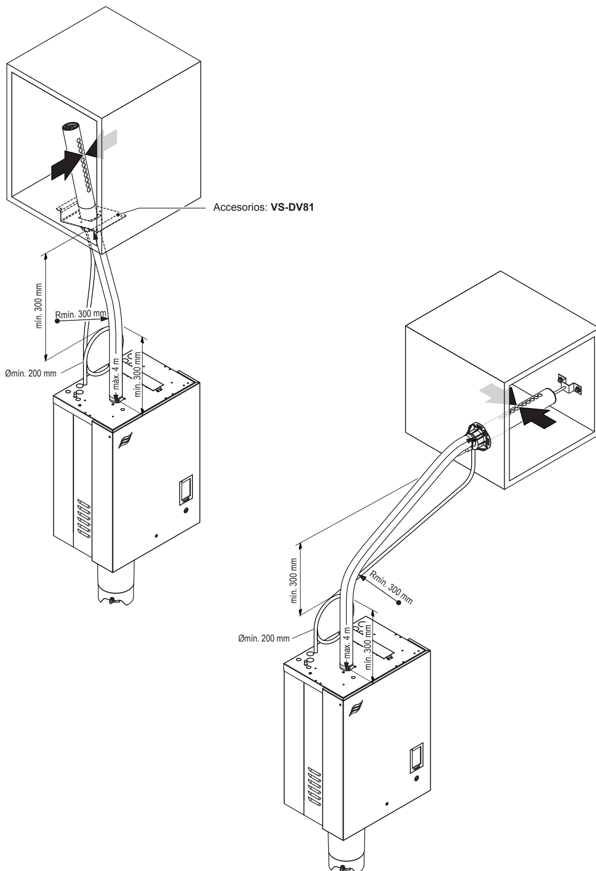
Fig. 18: El tubo de distribución de vapor está montado más de 500 mm por encima del borde superior del equipo.
