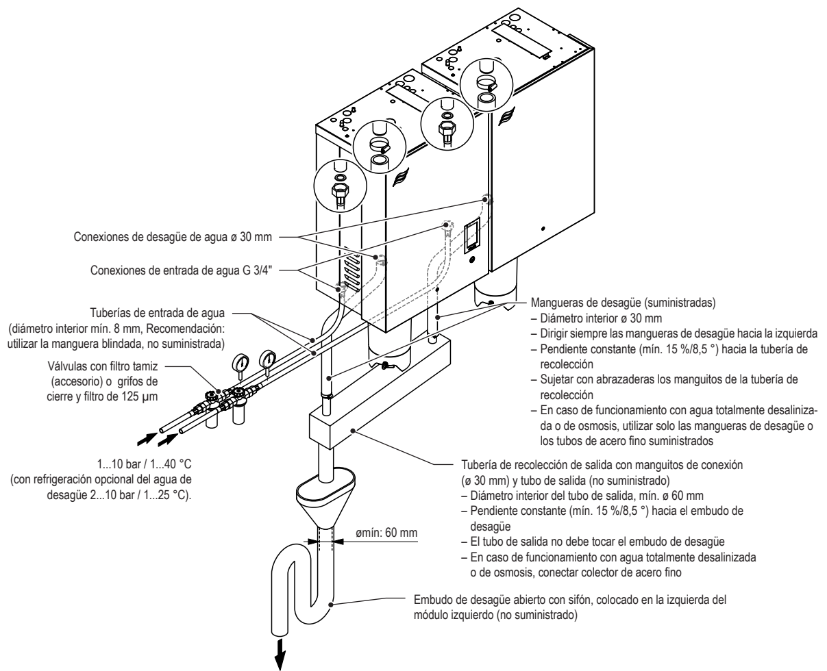
Fig. 24: Resumen de la instalación de agua para equipos dobles medianos ("M")
