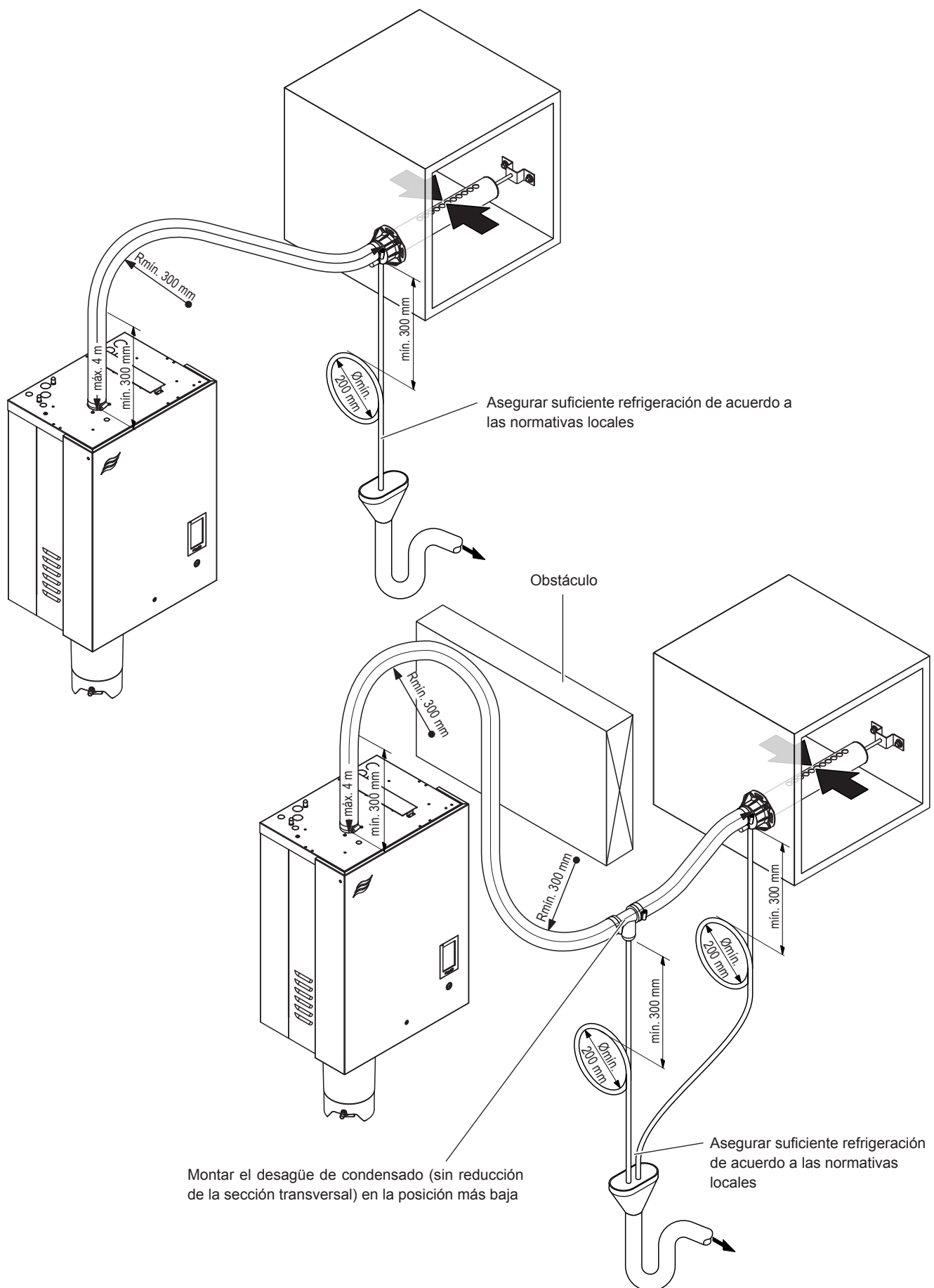
Fig. 19: El tubo de distribución de vapor está montado menos de 500 mm por encima o por debajo del borde superior del equipo.
